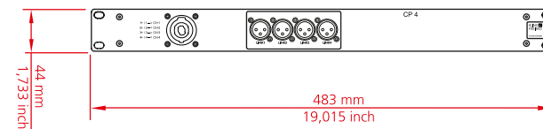
Connector Panel CP 4
