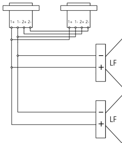
Verdrahtungsschema SW 215D
