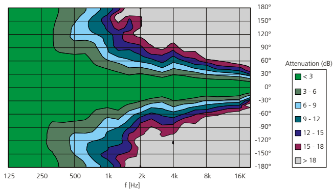
Horizontales Abstrahlverhalten
